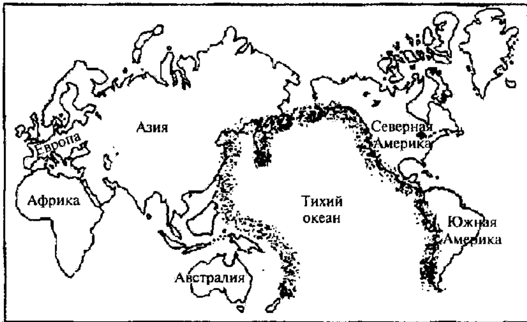
Рис. 1.10. Зоны землетрясений
