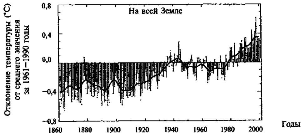
Рис. I.6. Средняя температура у поверхности Земли а) за последние 140 лет
