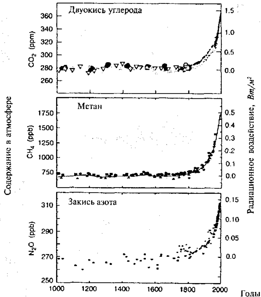
Рис. I.7. Содержание в атмосфере парниковых газов
