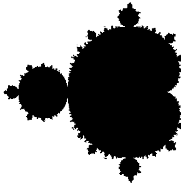
Рис. I.9. Множество Мандельброта
