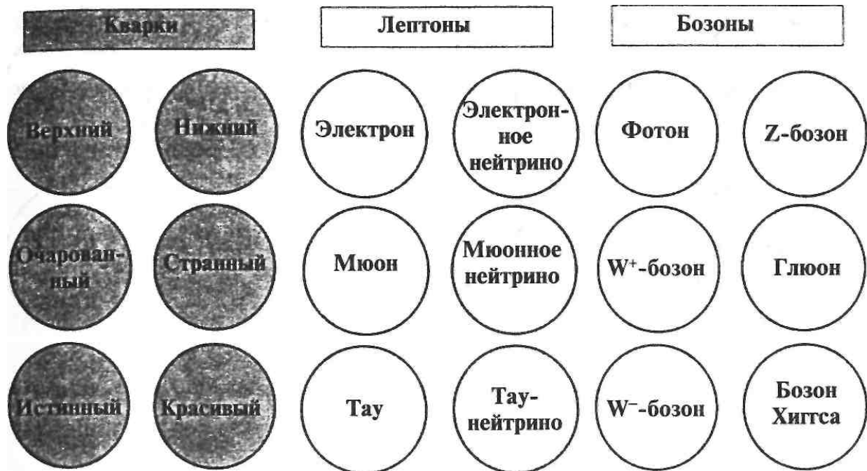
Рис. 2.5. Основные частицы
